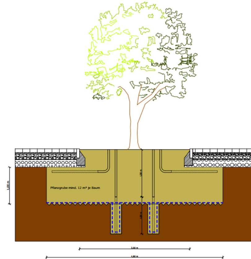
Längsschnitt Baumstandort
