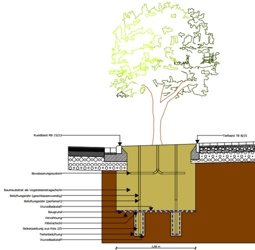
Querschnitt Baumstandort
